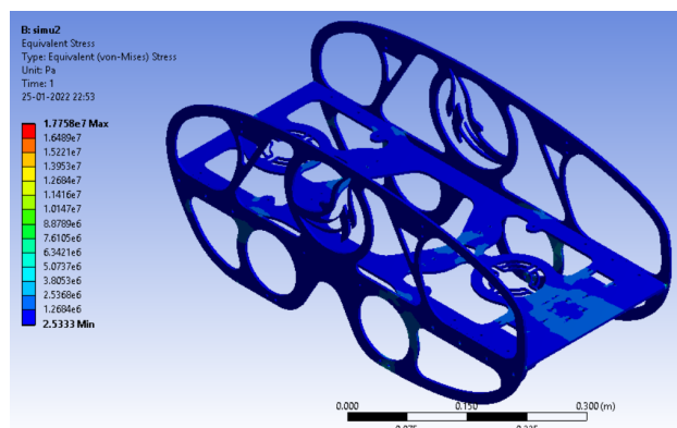
Von Mises Stress analysis of Arkaja 2.0 frame in Ansys
